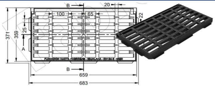
Grelha Sumidoura Anti-roubo C250 683x371x40 FAB.
