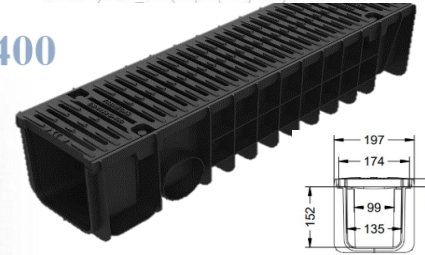
Canal PP c/ Grelha Fundição 200 MM D400
